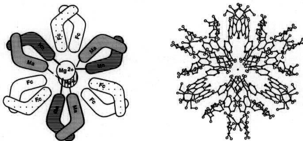
ツユクサの青色色素コンメリニン 会合模式図（左）とX線結晶解析図（右）
